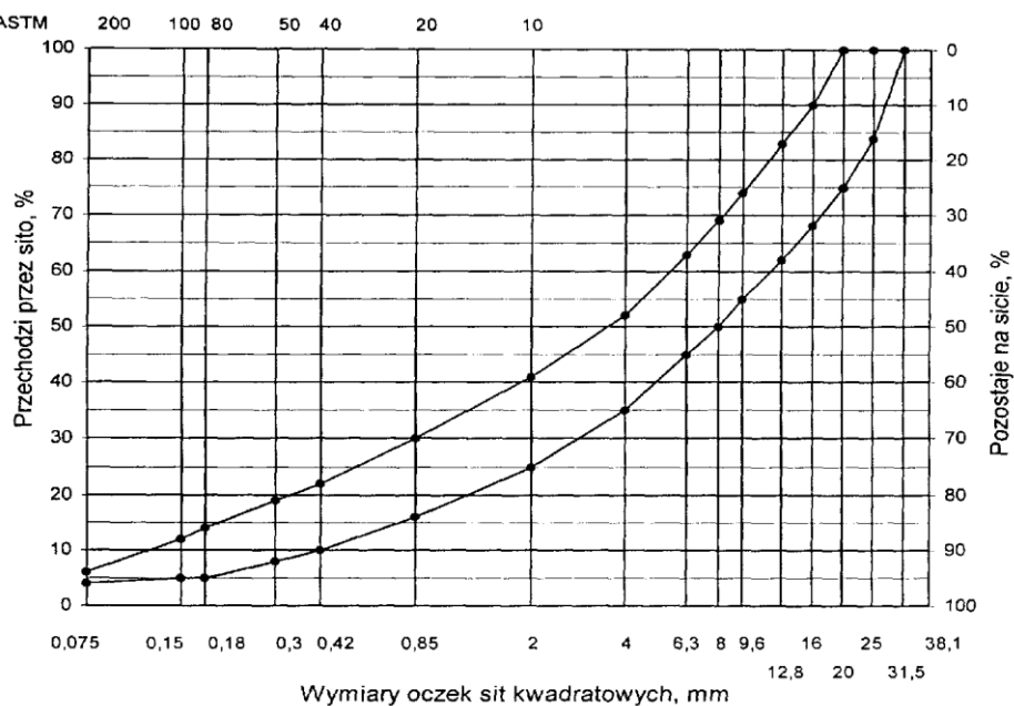
Rys. 2. Krzywe graniczne uziarnienia mieszanki mineralnej BA od 0 do 20 mm do warstwy wiążącej nawierzchni drogi o obciążeniu ruchem KR4
