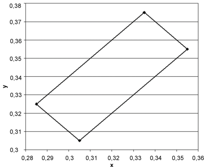
Rys. 1. Współrzędne chromatyczności x,y dla barwy białej oznakowania x,y dla barwy żółtej oznakowania
