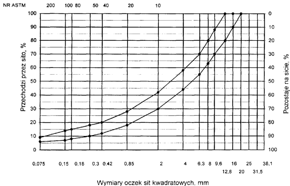
Rys. 1. Krzywe graniczne uziarnienia mieszanki mineralnej BA od 0 do 16 mm do warstwy ścieralnej nawierzchni drogi o obciążeniu ruchem KR4
