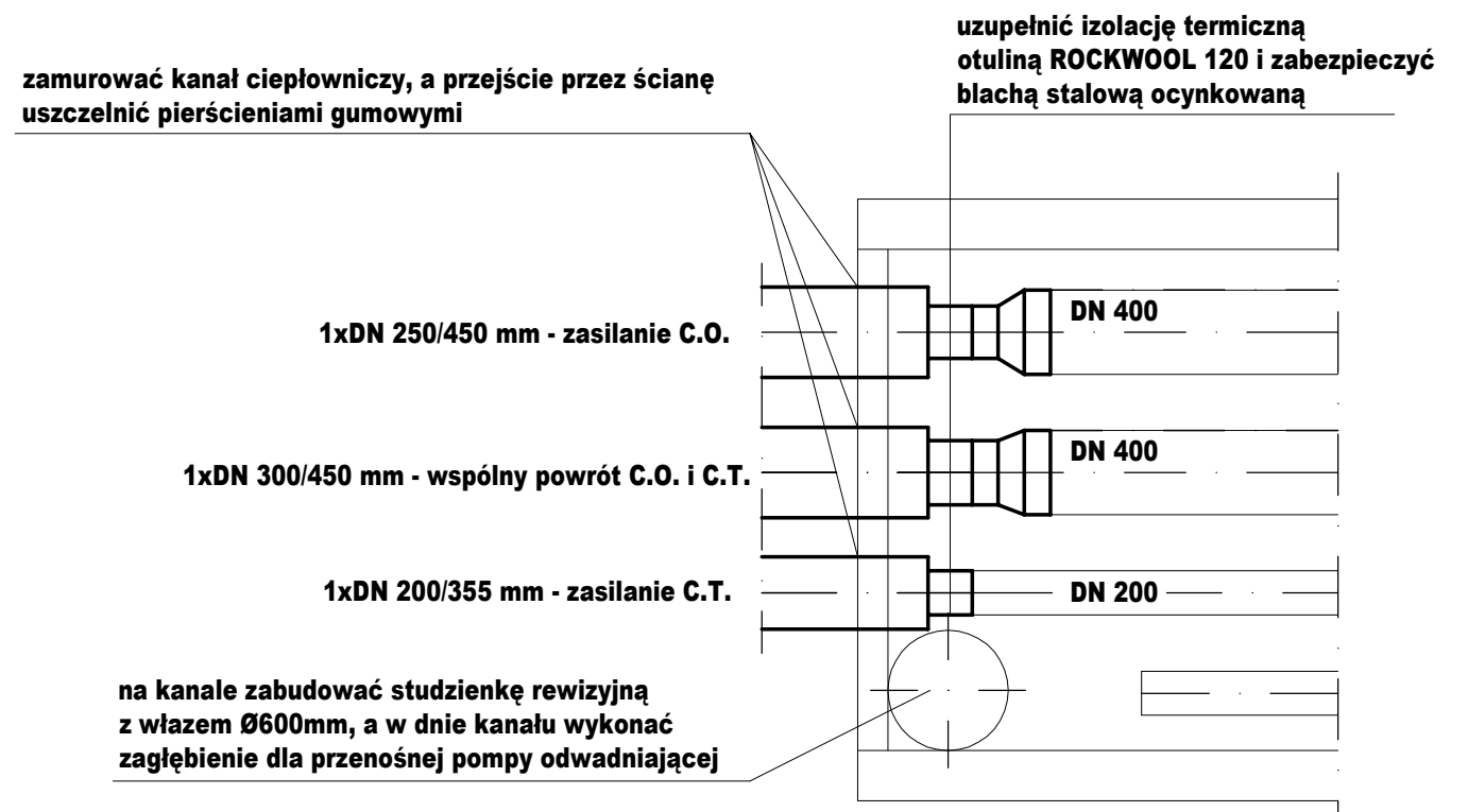
PUNKT "A" - szczegół
