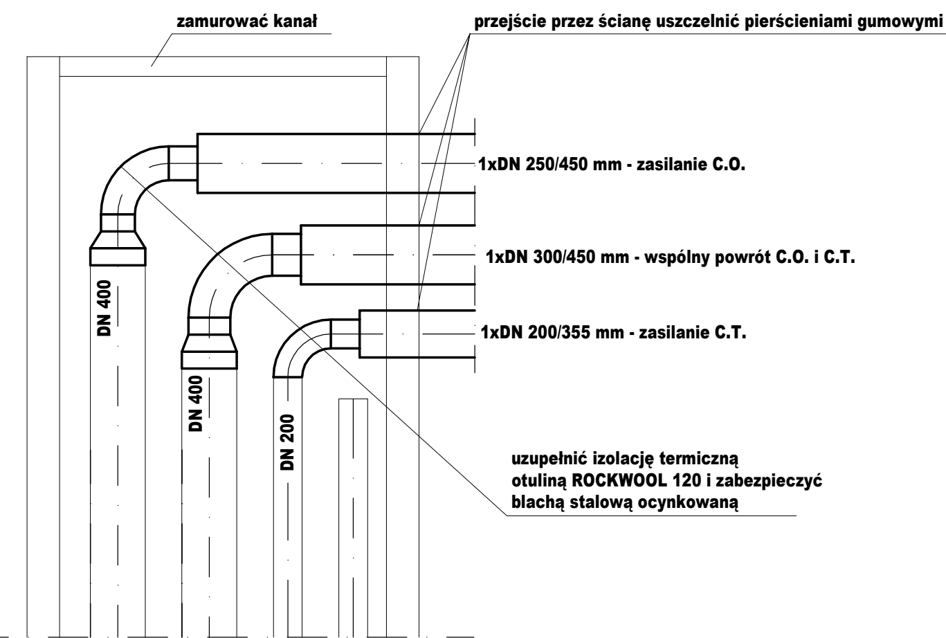
PUNKT "D" - szczegół
