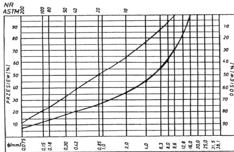
Rys. 1. Krzywe graniczne uziarnienia mieszanki mineralnej 0÷12,8 mm do warstwy ścieralnej z betonu asfaltowego dla KR 1-2
