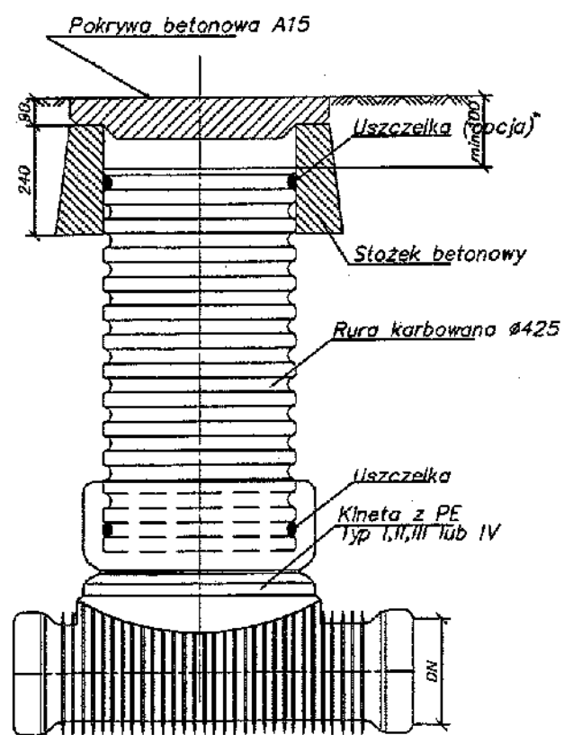
STUDZIENKA Ø425
