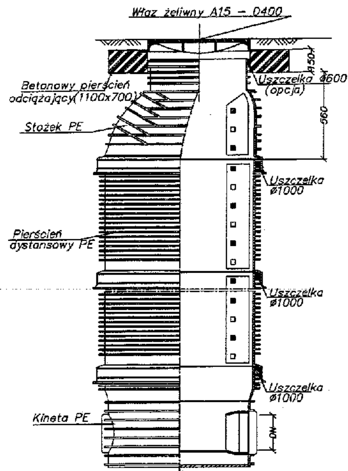
STUDZIENKA Ø1000
