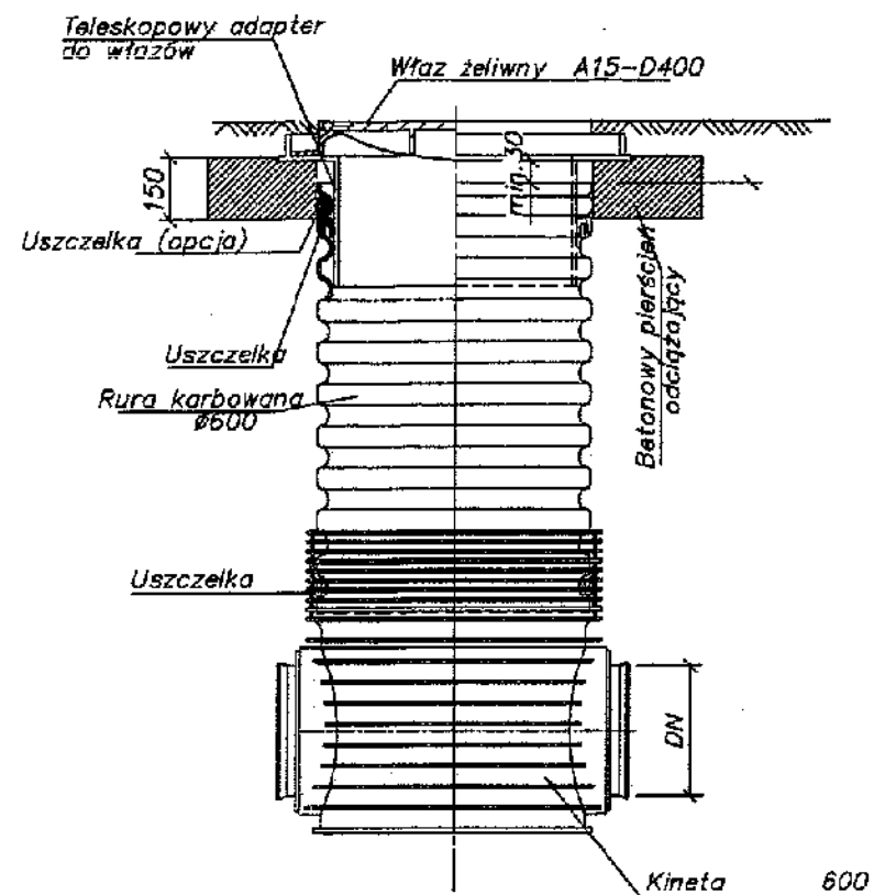
STUDZIENKA Ø600
