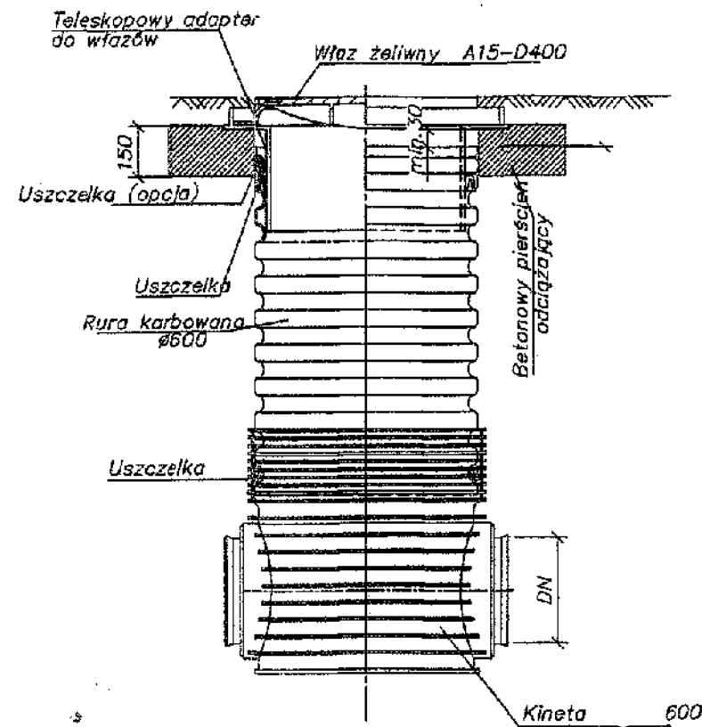
STUDZIENKA Ø 600
