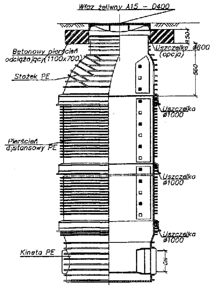
STUDZIENKA Ø 1000
