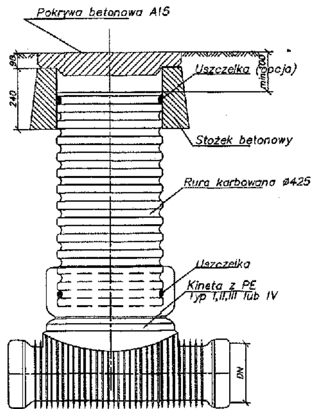
STUDZIENKA Ø 425
