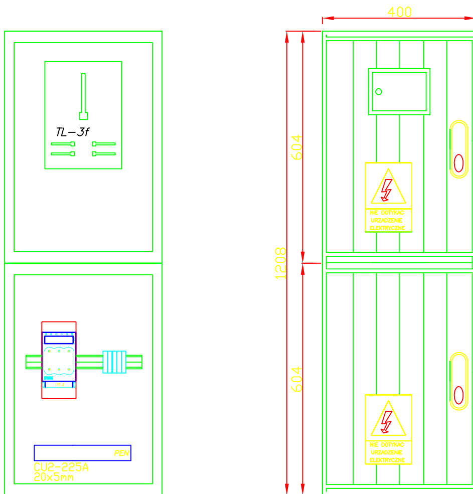
Układ pomiarowy bezpośredni typu ZPT
