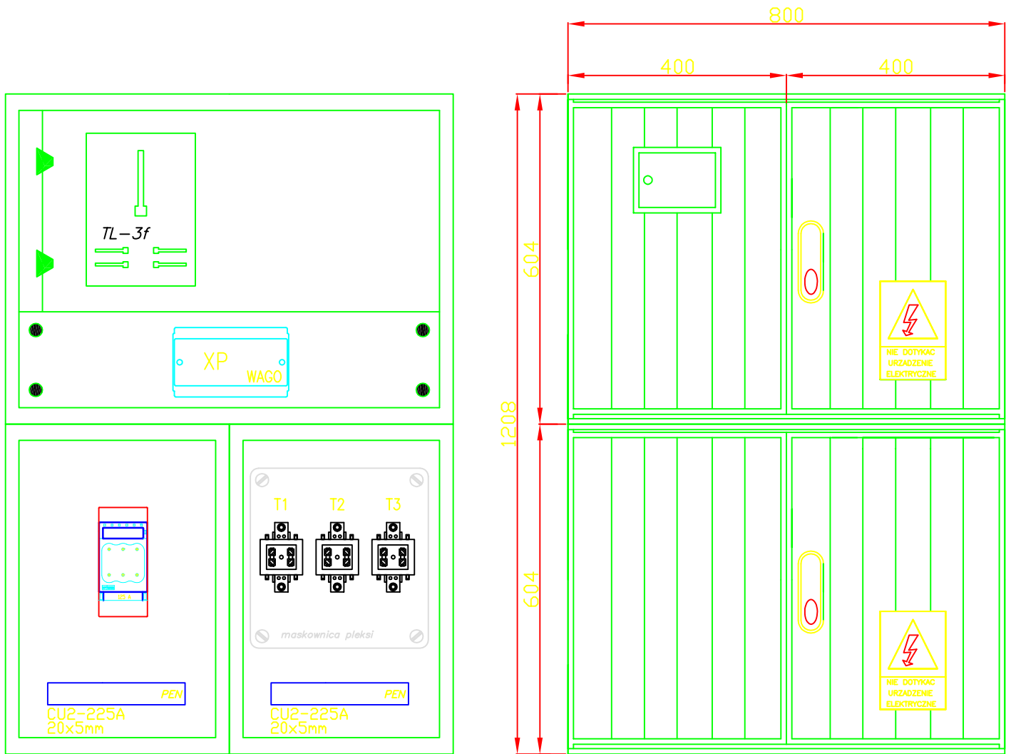
Układ pomiarowy półpośredni typu UP-2
