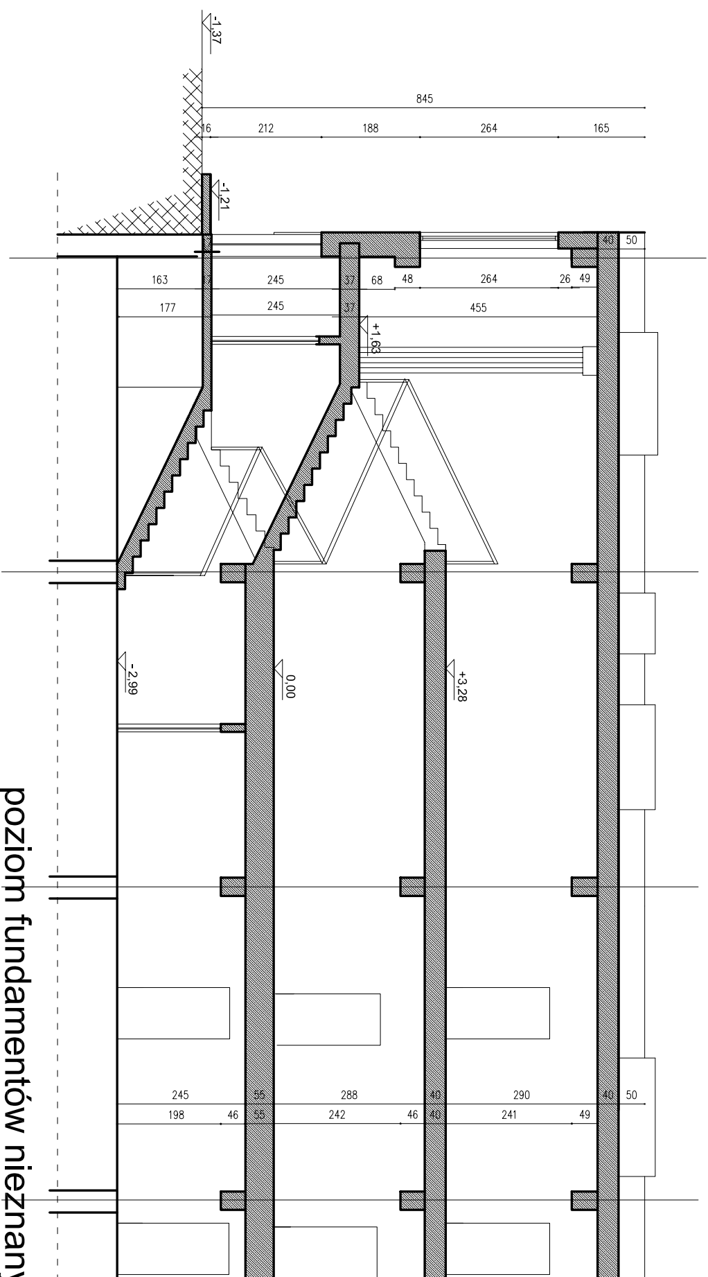
przekrój B-B
