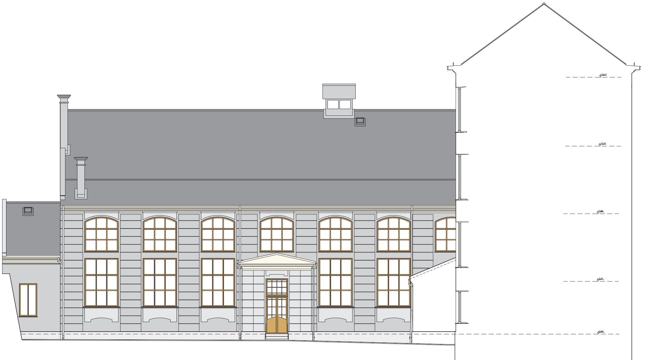
ELEWACJA SALI GIMNASTYCZNEJ OD STRONY Sp1
