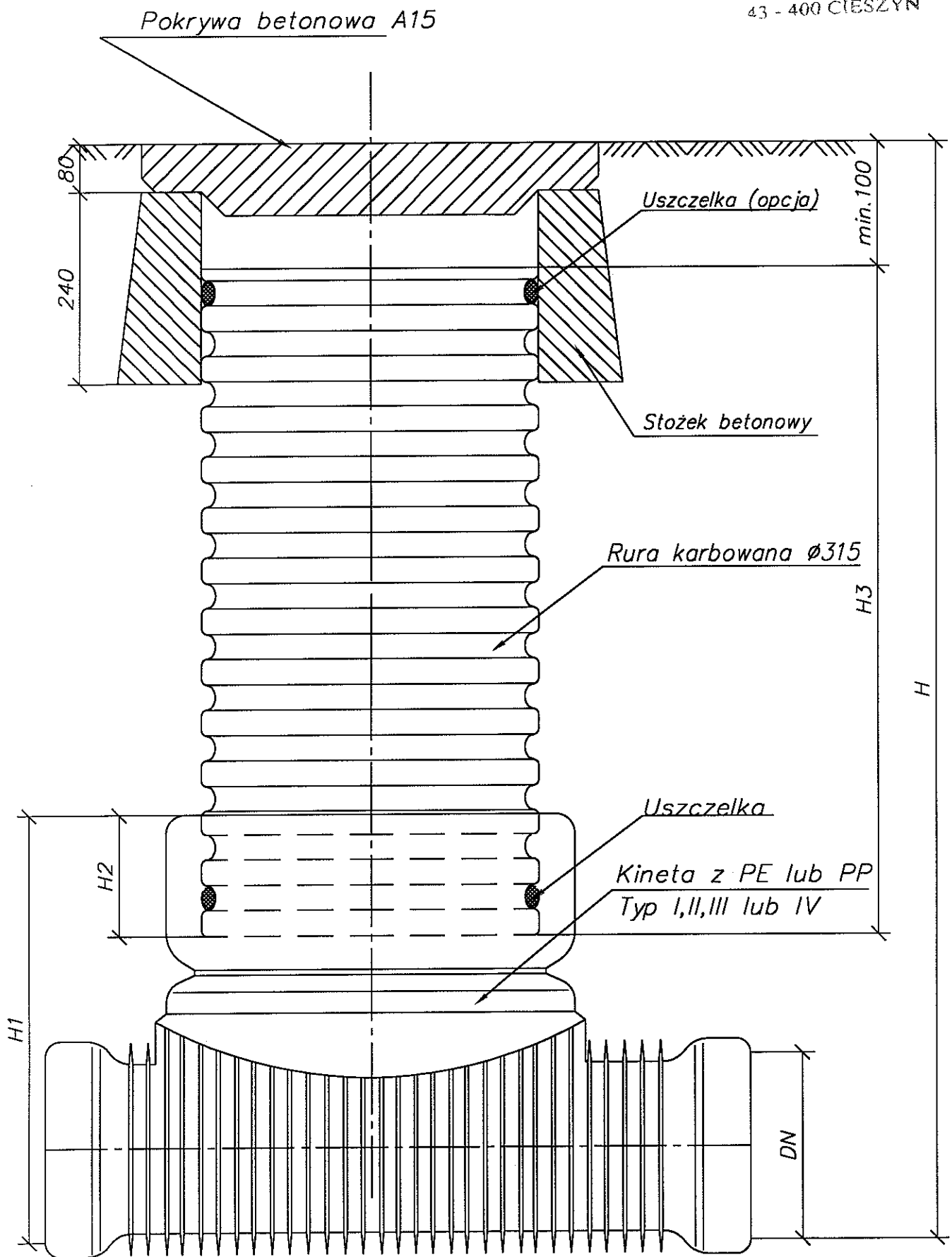
Studzienka kanalizacyjna \varnothing 315 niewłazowa
