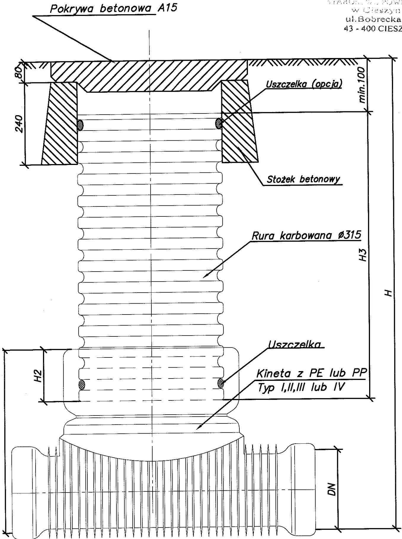
Studzienka kanalizacyjna \phi 315 niewłazowa
