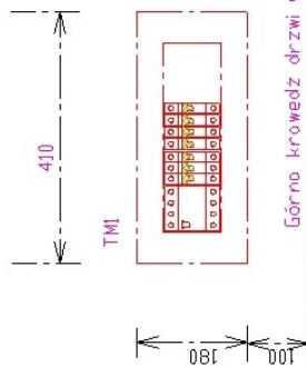
Schemot i widok tablicy TM
