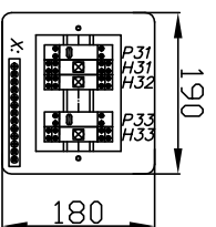
Tablica sterowania oświetleniem boisk TSOB
