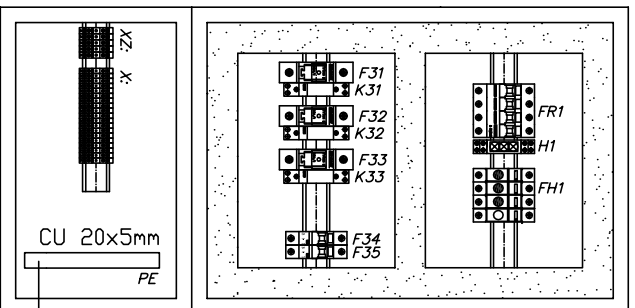
Tablica oświetlenia boisk TOB
